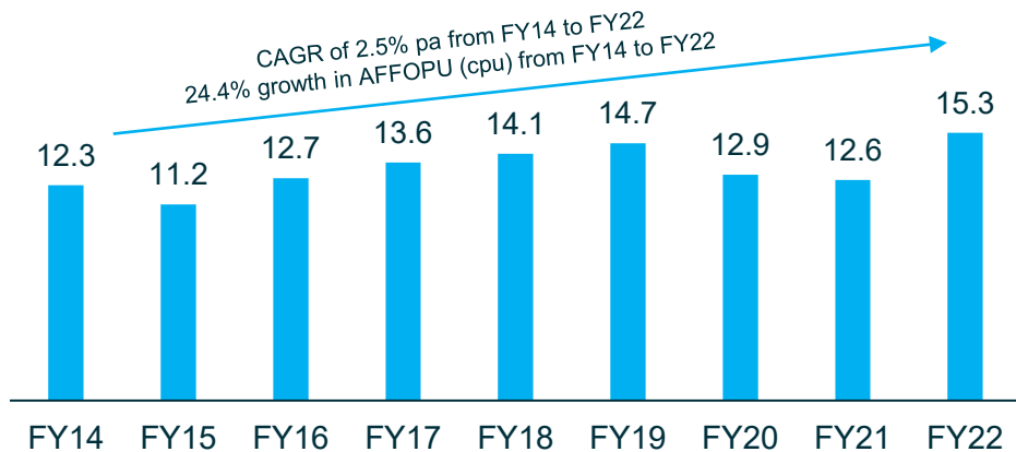
AFFOPU (cpu)
